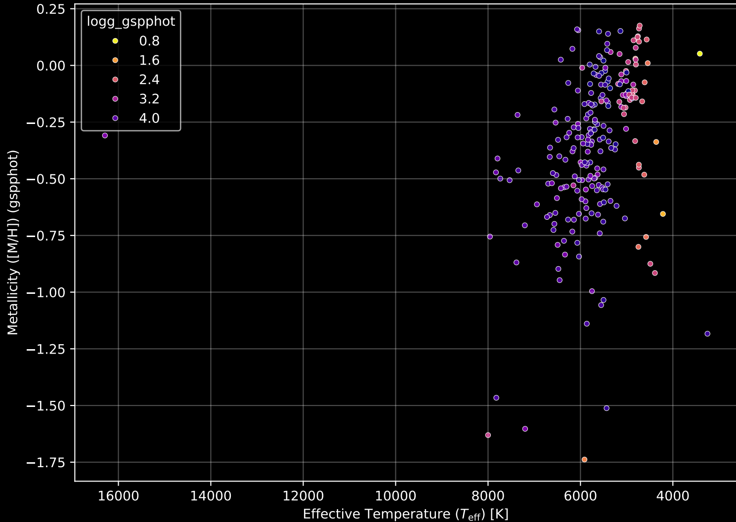
GALAH DR4 Field: [7170] Stellar Population Parameters (n= 229)
